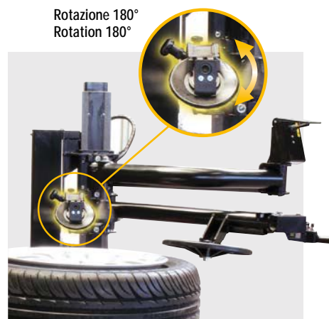
PLUS83S PLUS83 con disco inclinato 45° PLUS83 with 45° tilted roller PLUS83 mit 45° geneigte Rolle PLUS83 avec rouleau incliné 45° PLUS83 con rodillo inclinado 45°
