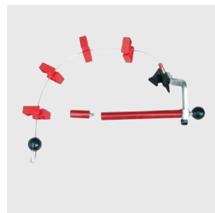
G1000A56 - 22" Premitalone 22" con trazione. 22" bead pushing device with pulling system. Wulstboy 22" mit Zugvorrichtung. Pousse-talon 22" avec traction. Prensa talón 22" con tracción.
